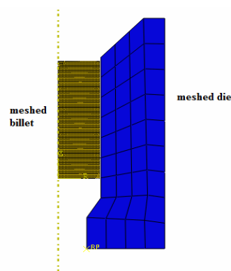
Fig. 3. FEM model
