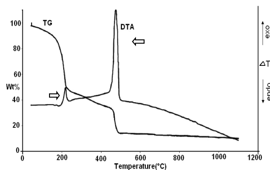
Fig. 1. STA trace of the gel.
