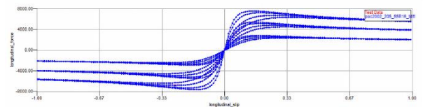
Figure22: Longitudinal Force Vs Longitudinal Slip
